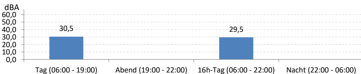
Abb. 9: LEQ bei Pistenbetriebsrichtung "östliche Winde" 157 Stunden im Messzeitraum
