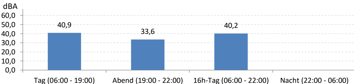
Abb. 8: LEQ bei Pistenbetriebsrichtung "Windstille" 219 Stunden im Messzeitraum
