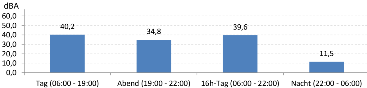
Abb. 7: LEQ bei Pistenbetriebsrichtung "westliche Winde" 441 Stunden im Messzeitraum
