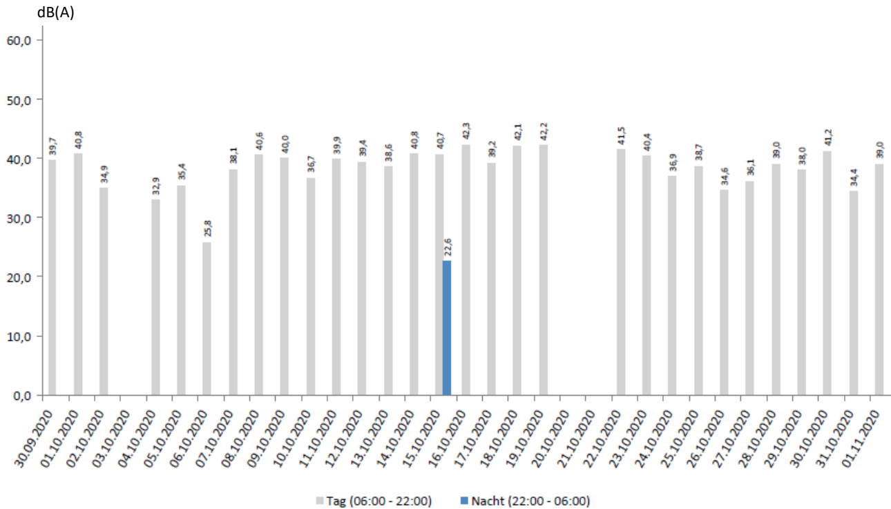
Abb.10: LEQ für Flugverkehr über den Messzeitraum
