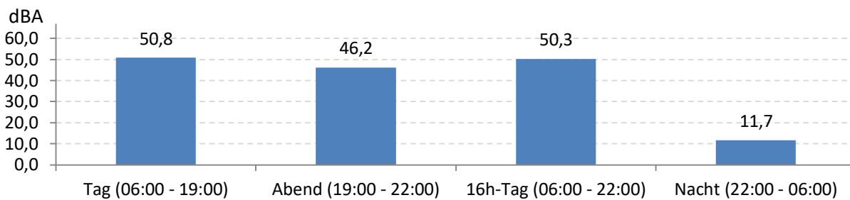
Abb. 7: LEQ bei Pistenbetriebsrichtung "westliche Winde"
