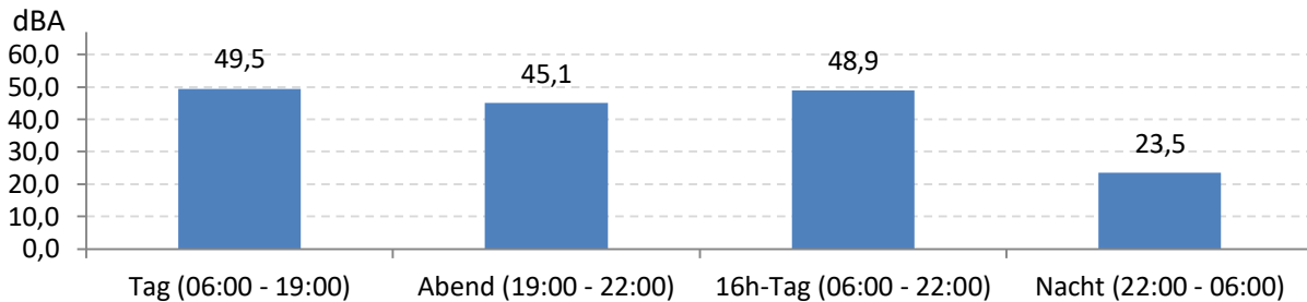
Abb. 6: LEQ für den gesamten Messzeitraum während der Messdauer (Gesamt: 720 Stunden)
