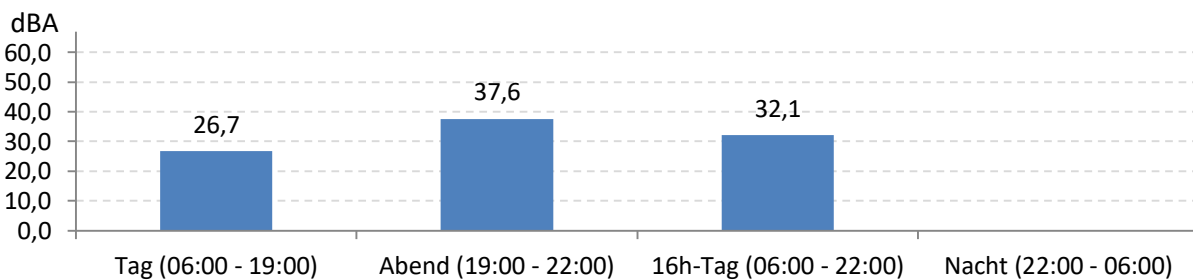
Abb. 8: LEQ bei Pistenbetriebsrichtung "Windstille"
