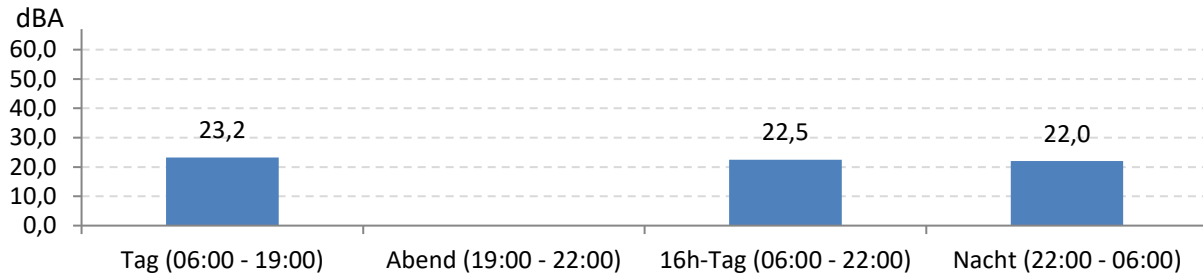
Abb. 7: LEQ bei Pistenbetriebsrichtung "westliche Winde" 379 Stunden im Messzeitraum
