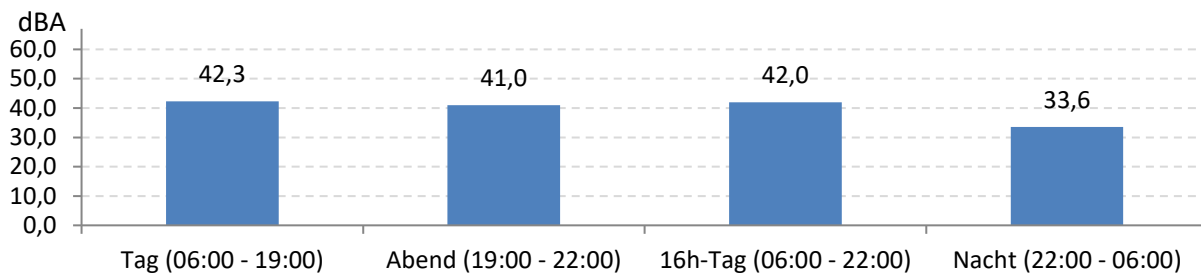
Abb. 9: LEQ bei Pistenbetriebsrichtung "östliche Winde" 136 Stunden im Messzeitraum
