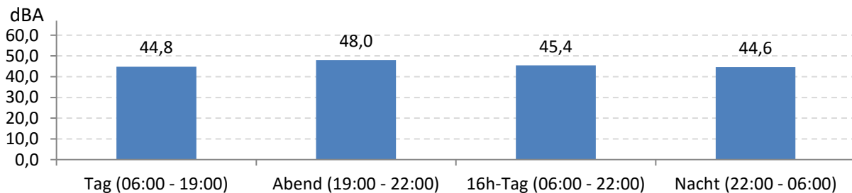
Abb. 8: LEQ bei Pistenbetriebsrichtung "Windstille" 202 Stunden im Messzeitraum
