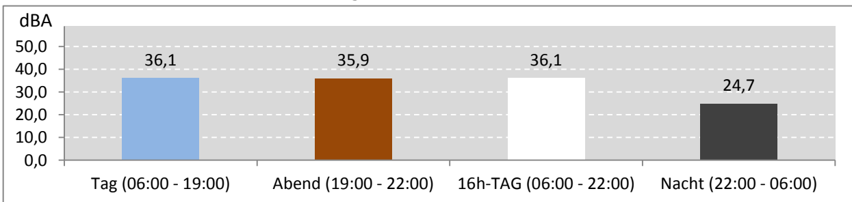
Abb. 8: LEQ bei Pistenbetriebsrichtung "Windstille" 160 Stunden im Messzeitraum
