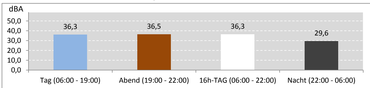
Abb. 7: LEQ bei Pistenbetriebsrichtung "westliche Winde" 231 Stunden im Messzeitraum
