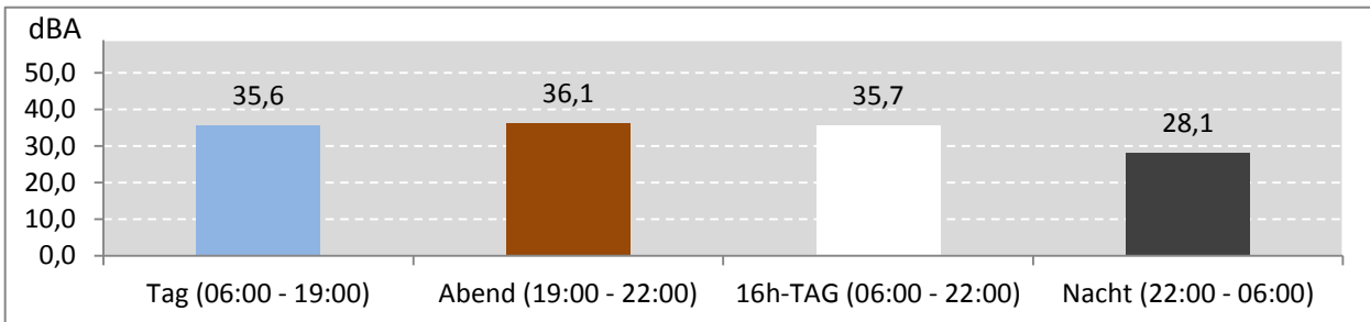
Abb. 6: LEQ für den gesamten Messzeitraum während der Messdauer (Gesamt: 532 Stunden)
