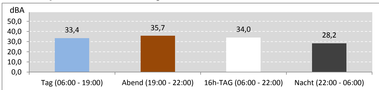
Abb. 9: LEQ bei Pistenbetriebsrichtung "östliche Winde" 141 Stunden im Messzeitraum
