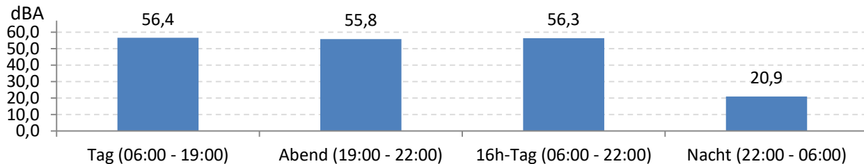
Abb. 7: LEQ bei Pistenbetriebsrichtung "westliche Winde"
