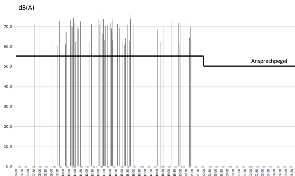
Abb. 13: Verteilung des Maximalpegels bei östlichen Winden
