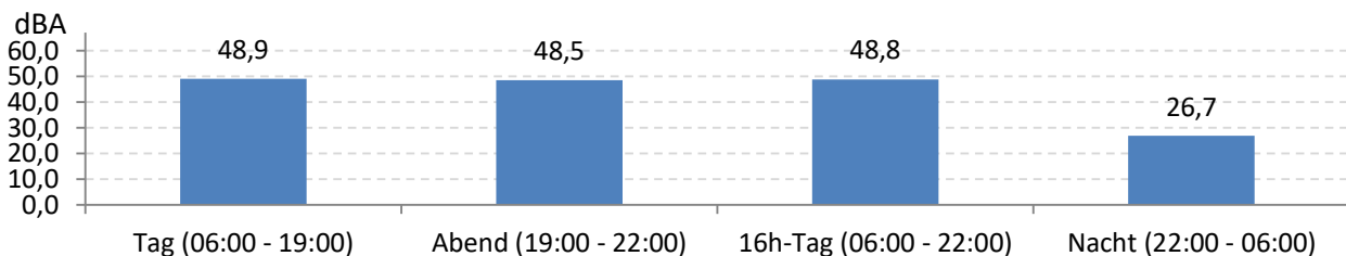
Abb. 8: LEQ bei Pistenbetriebsrichtung "Windstille"
