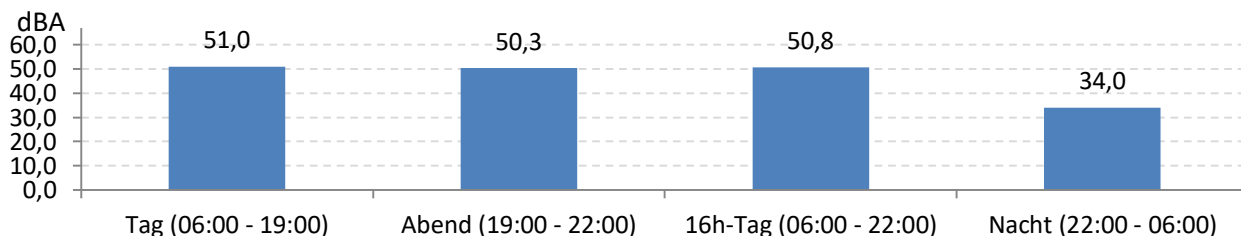
Abb. 9: LEQ bei Pistenbetriebsrichtung "östliche Winde"
