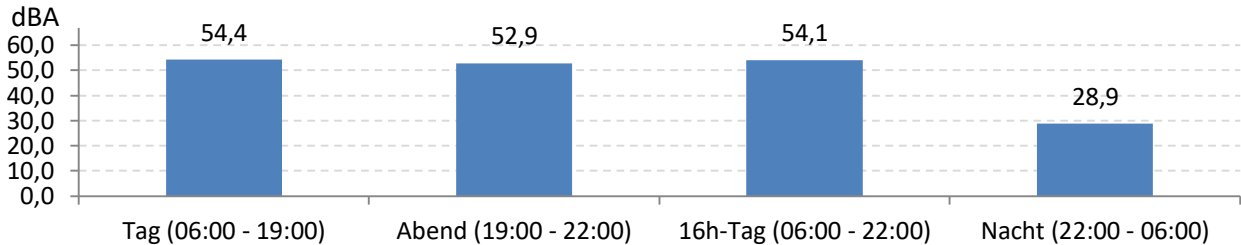
Abb. 6: LEQ für den gesamten Messzeitraum während der Messdauer (Gesamt: 720 Stunden)
